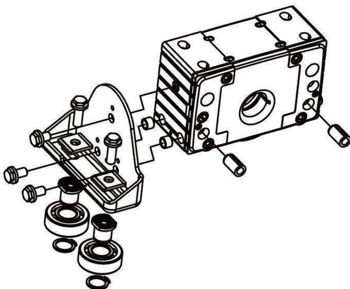
DRS112-200 Horizontal guide rollers
