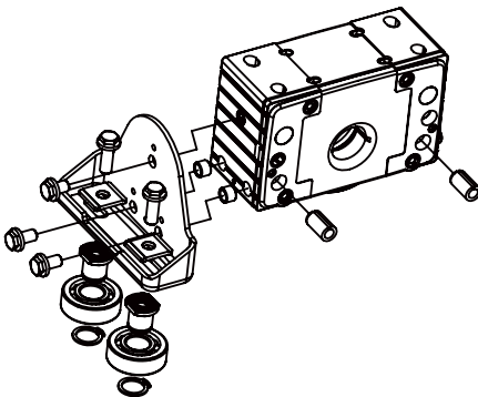
DRS112-200 Horizontal guide rollers
